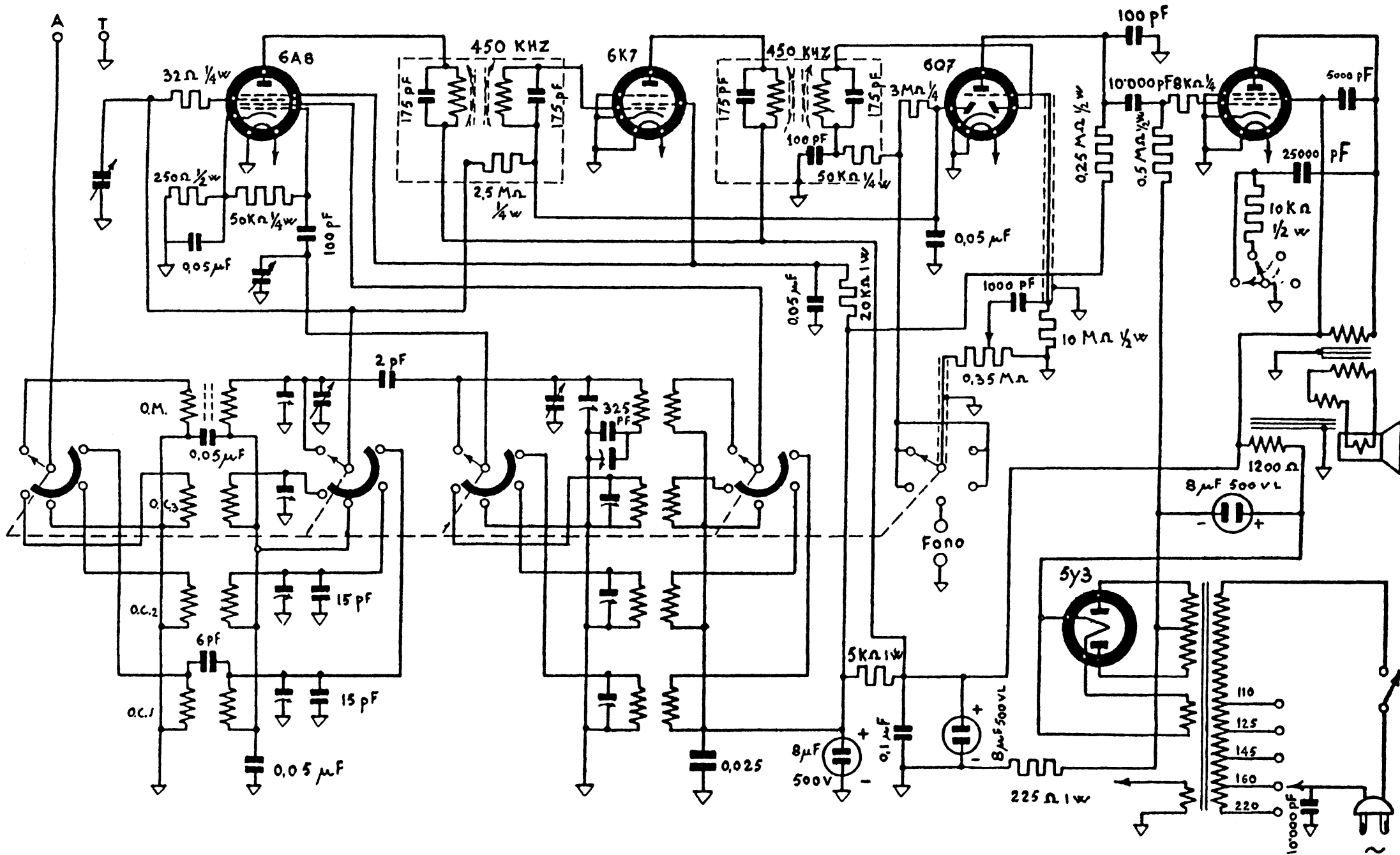
14 - FARA RADIO - MOD. D 541. Gamme: da 188 a 572 m, da 13 a 22 m, da 22 a 35 m, da 35 a 63 m. Media frequenza: 450 kc/s. Tensioni placca: 260 V; al catodo della 5Y3 G 300 V. Placca oscillatrice: 200 V. Potenza: 4 watt circa. Produzione 1945-46.
